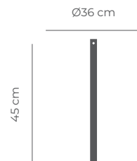
Poste LINE MINI Esc. 1:20 (Peso: 6kg)
