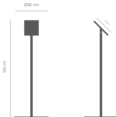
Poste atril LINE A5
