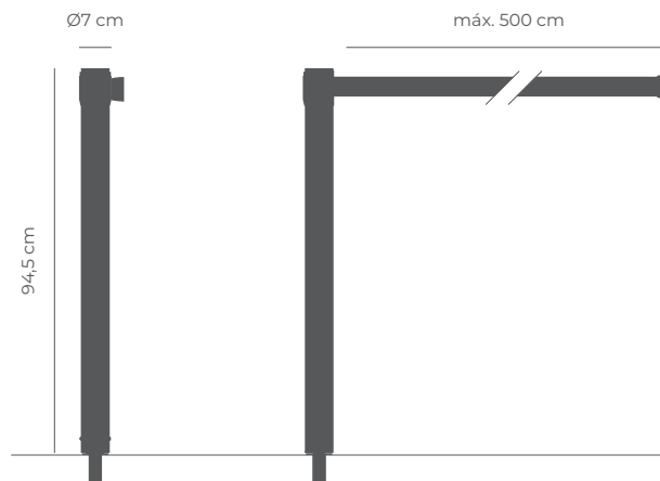
Poste UNFIX Esc. 1:20 (Peso: 4kg)
