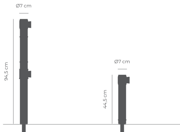
Poste UNFIX DUAL Esc. 1:20 (Peso: 4Kg)
