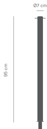
Poste Classic Unfix Esc. 1:20 (Peso: 2 kg)
