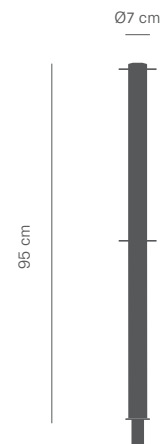
Poste Classic Unfix Dual Esc. 1:20 (Peso: 2 kg)
