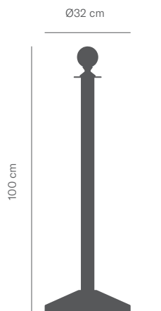
Poste GOLD Esc. 1:20 (Peso: 9kg)
