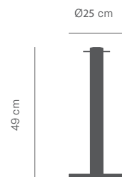
Poste Classic Fix Mini Esc. 1:20 (Peso: 1,5 kg)
