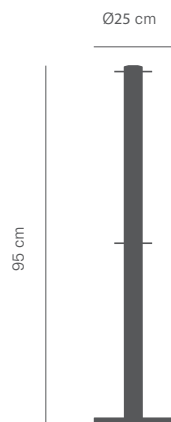
Poste Classic Fix Dual Esc. 1:20 (Peso: 2,5 kg)
