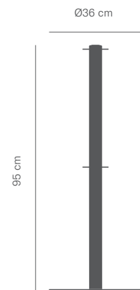
Poste Classic Dual Esc. 1:20 (Peso: 7 kg)
