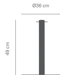
Poste Classic Mini Esc. 1:20 (Peso: 6kg)
