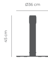
ECO MINI post Esc. 1:20 (Weight: 4kg)
